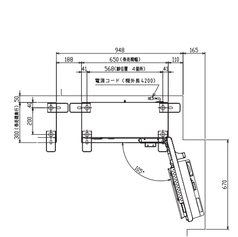
設置寸法図 (単位：mm)
